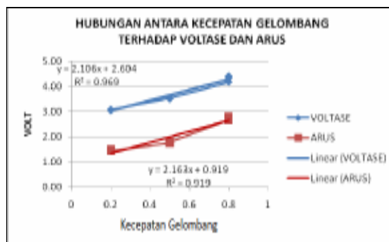
Gambar 8. Grafik pengaruh kecepatan gelombang terhadap Arus dan Voltase
